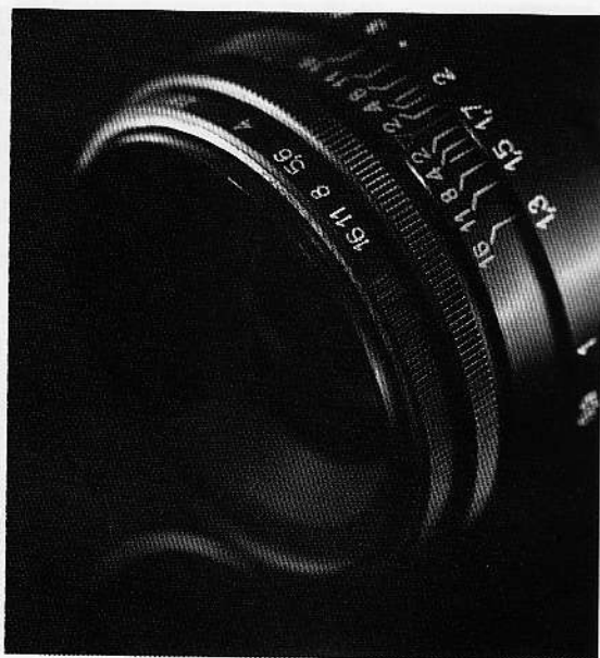
Sessant'anni e più. Nel 1954 le industrie fotografiche adottarono una definizione di valore di esposizione.
